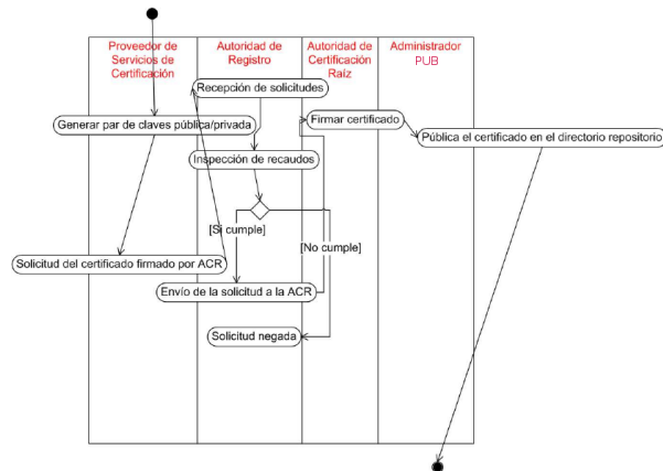
Figura 5.6 Diagrama de actividades para el caso de uso “Emisión de Certificados”
