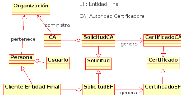
Figura 5.5 Diagrama de clases
