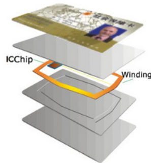
Figura 1.12 Tarjeta sin contacto.
