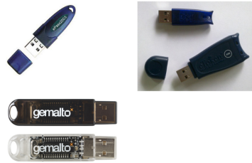
Figura 1.9 Tokens criptográficos.
